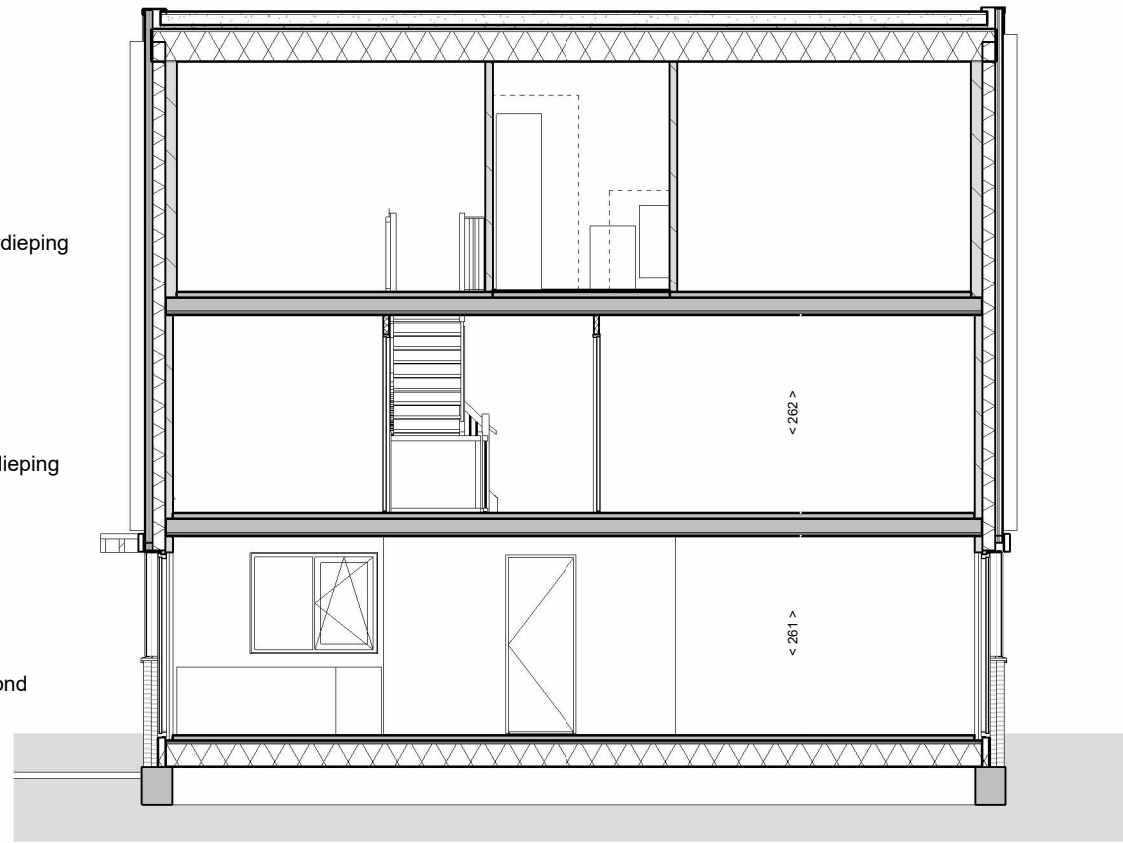
dwarsdoorsnede
