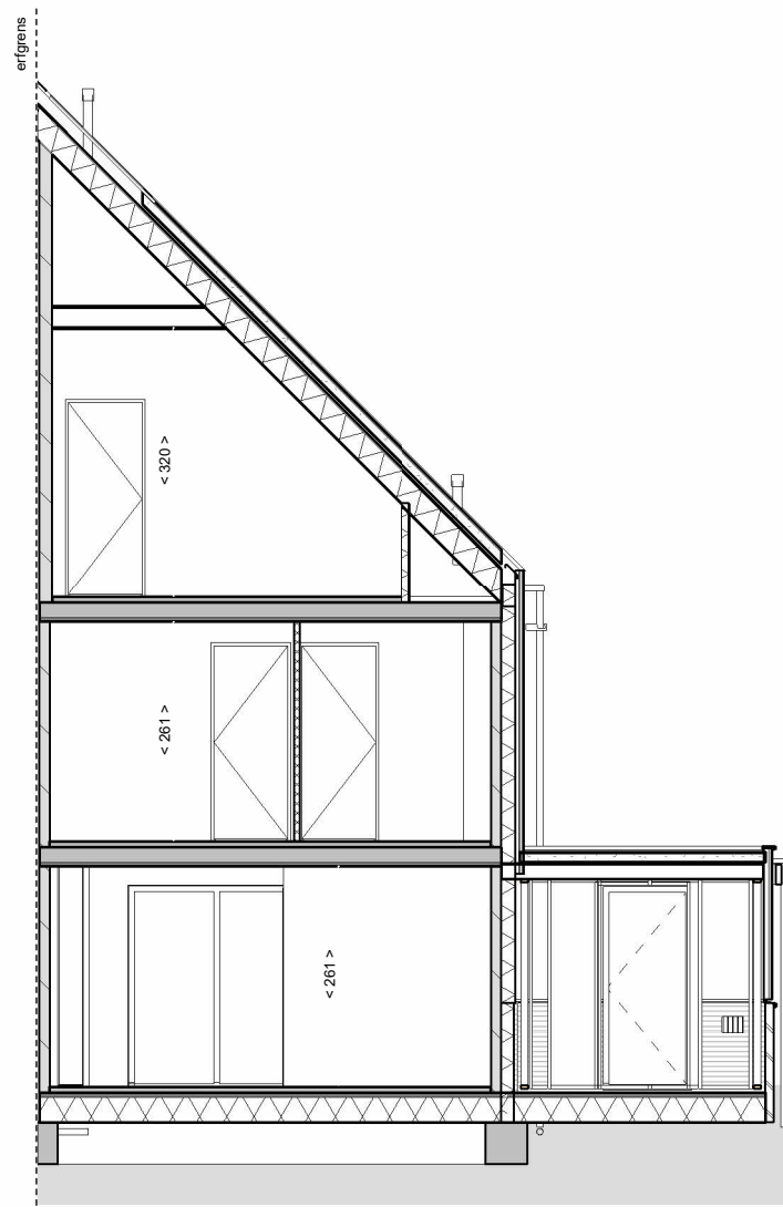
langsdoorsnede
