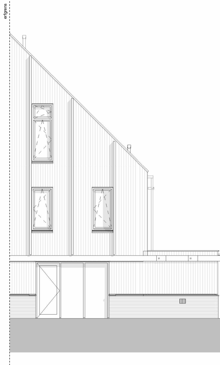
achtergevel (noordoost)
