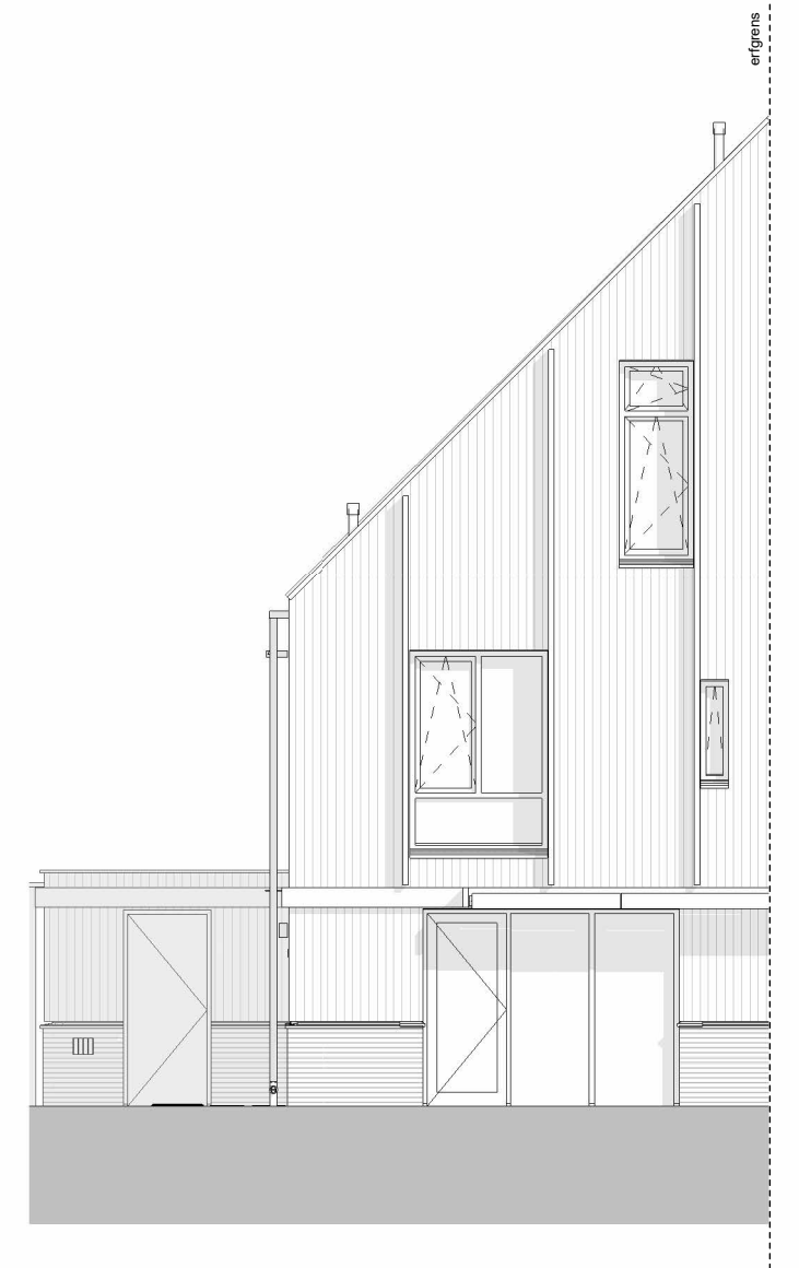
voorgevel (zuidwest)
