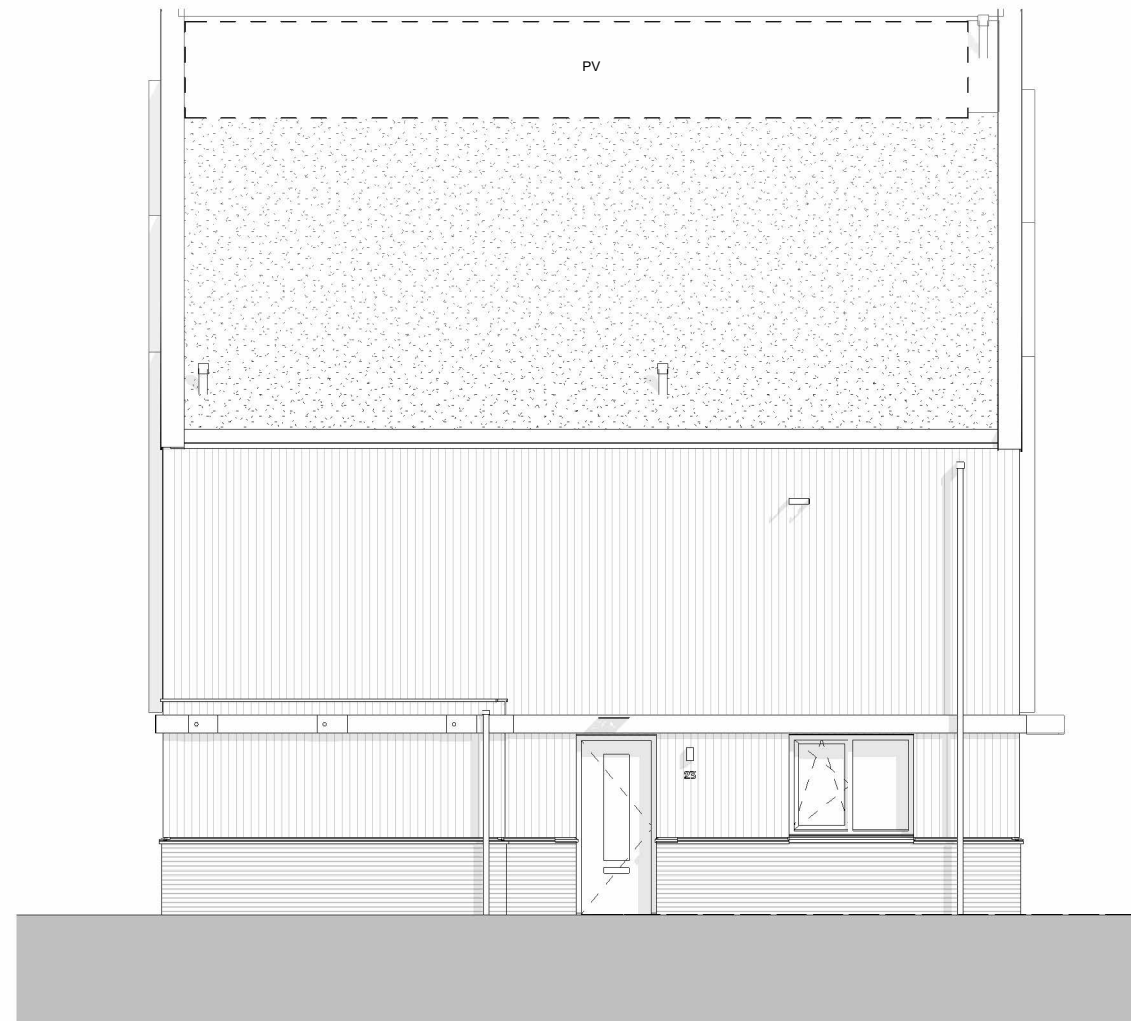
zijgevel (noordwest)
